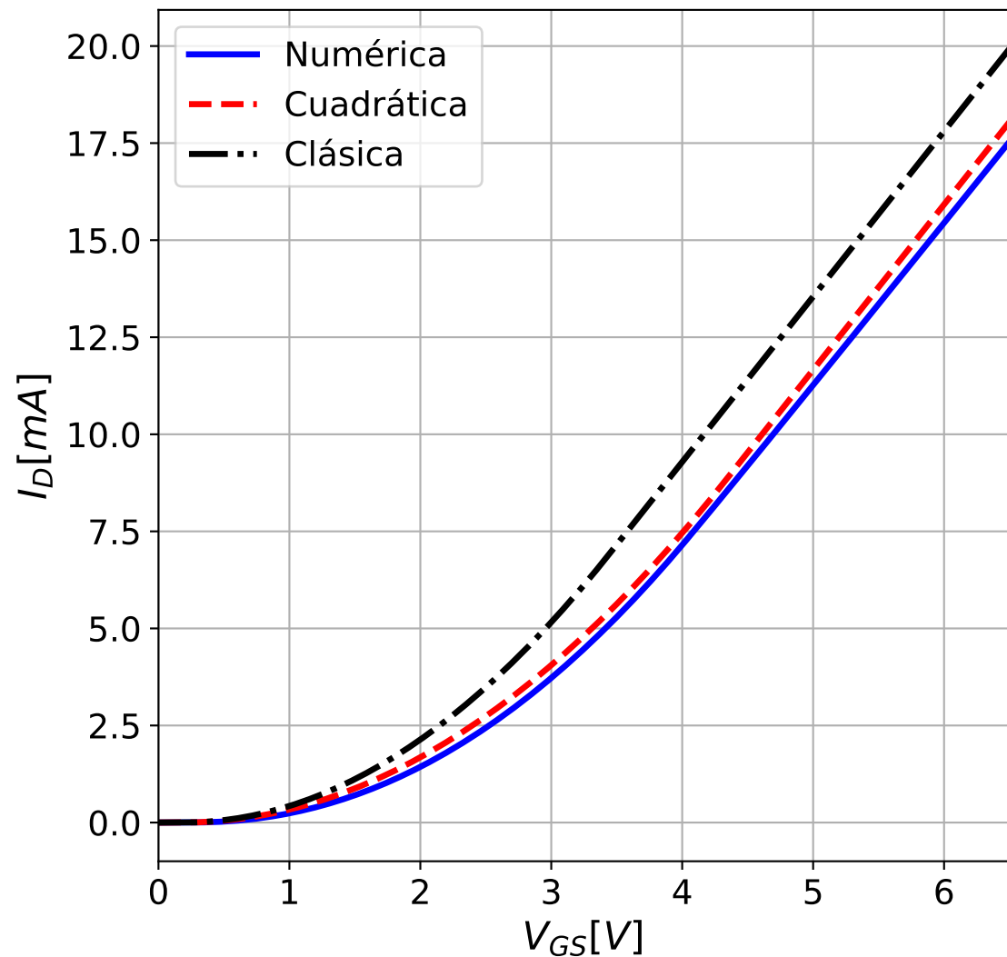
Curva de transferencia para V_{DS} = 0,5 \cdot V_{DD} = 3.25 V
